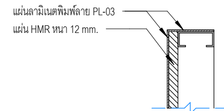
ขยายผนัง 9 มาตราส่วน 1 : 5
