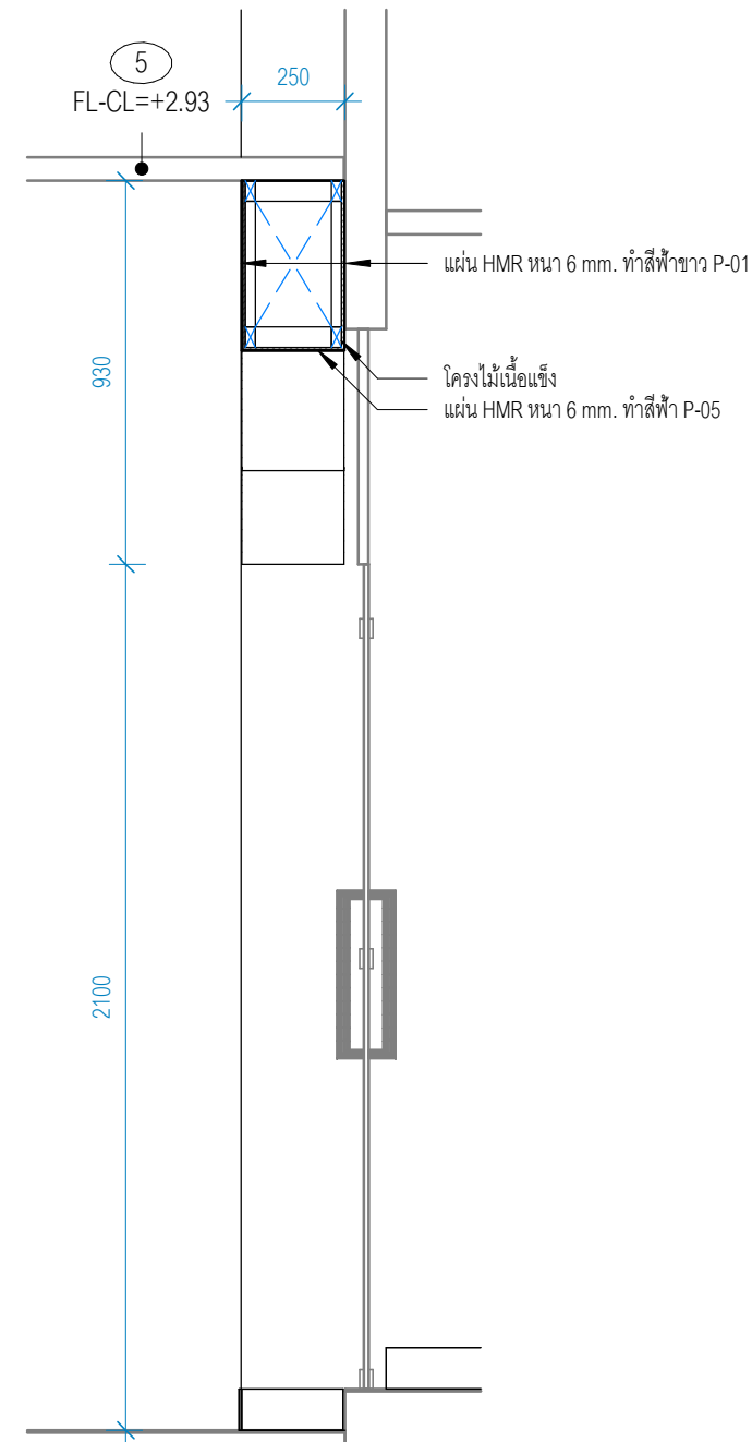
รูปตัด A' ขยายชั้มประตู มาตราส่วน 1 : 20
