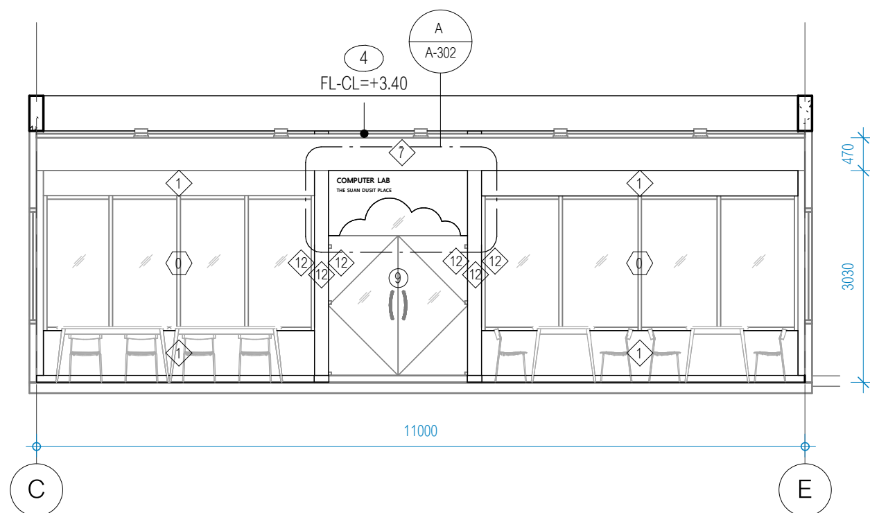
รูปด้าน 15
