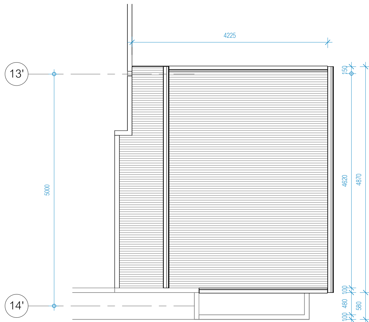
ผังหลังคาส่วนต่อเติม มาตราส่วน 1 : 50
