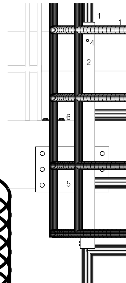
Detail B มาตราส่วน 1 : 10
