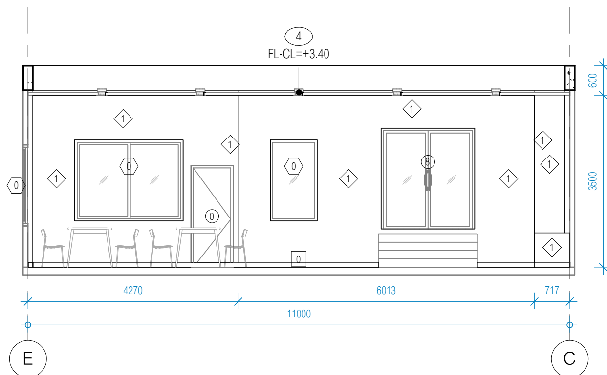
รูปด้าน 13
