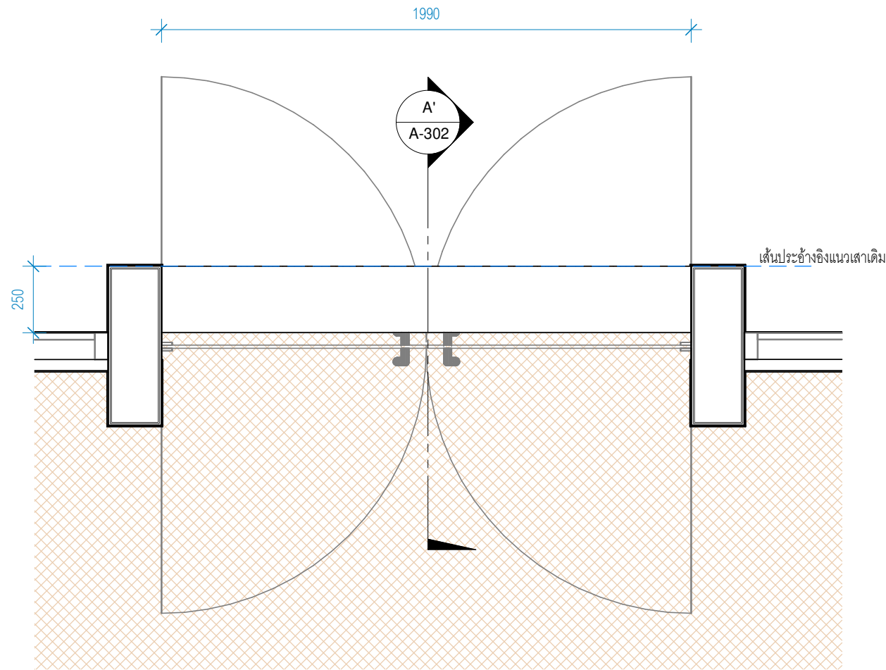
ผังแบบขยายชั้มประตู A มาตราส่วน 1 : 20
