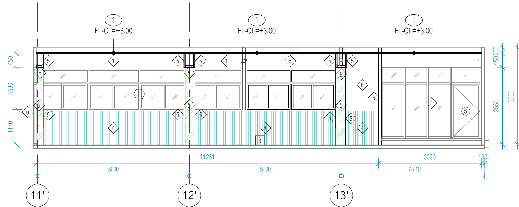
รูปด้าน 6
