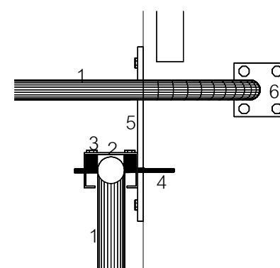
Detail A มาตราส่วน 1 : 10
