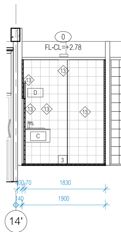
WC1 รูปด้าน 1 มาตราส่วน 1 : 50
