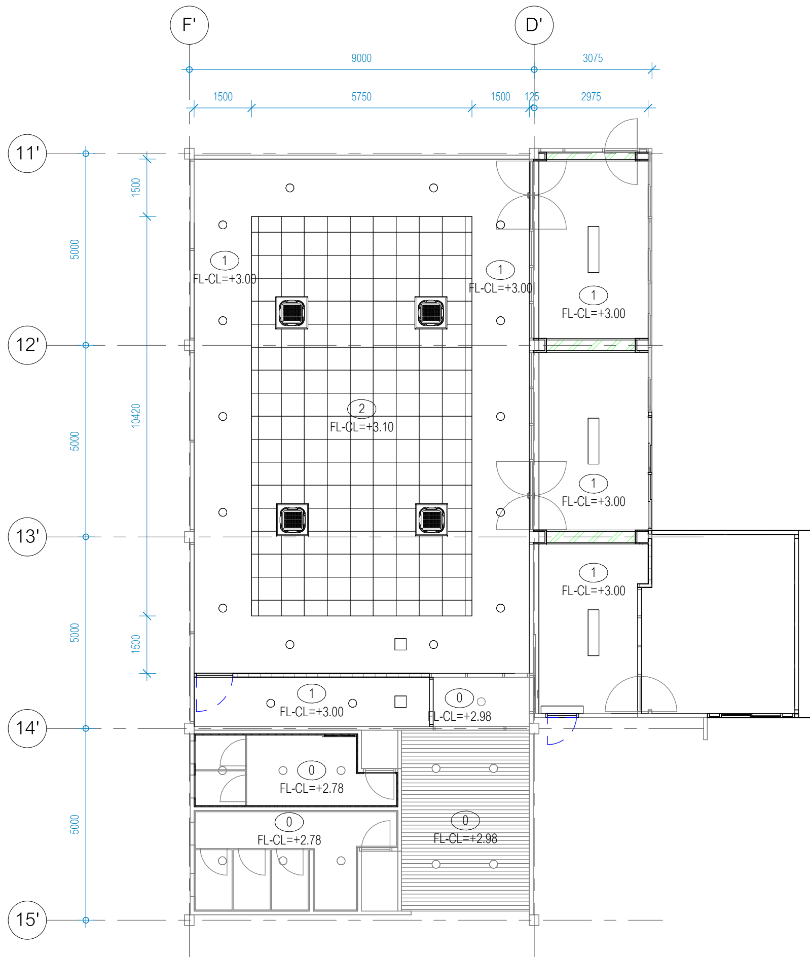
ผังฝ้าห้อง Lecture room มาตราส่วน 1 : 100
