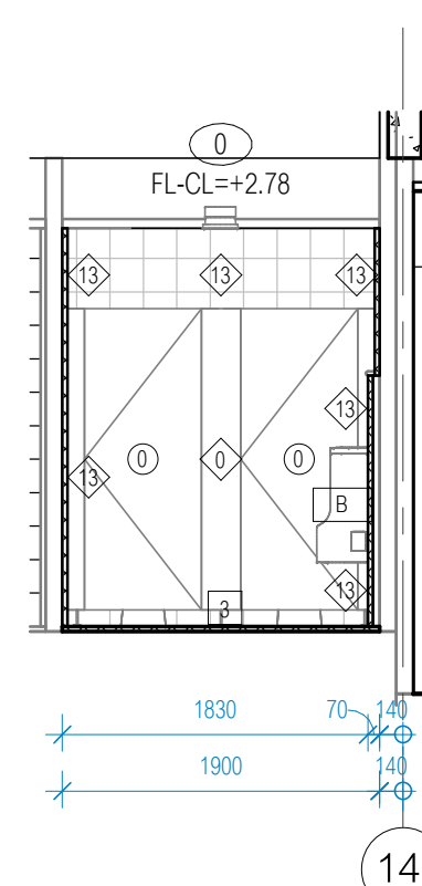
WC1 รูปด้าน 3 มาตราส่วน 1 : 50
