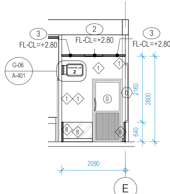
รูปด้าน 24 มาตราส่วน 1 : 75
