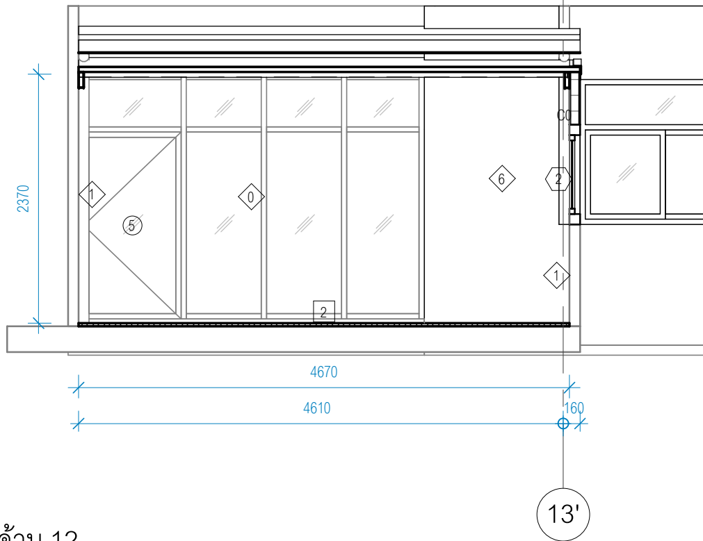
รูปด้าน 12 มาตราส่วน 1 : 50
