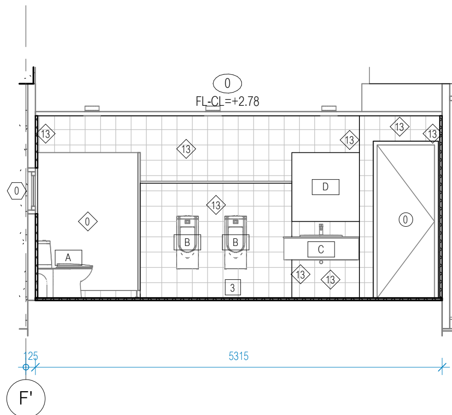
WC1 รูปตัด 4 มาตราส่วน 1 : 50
