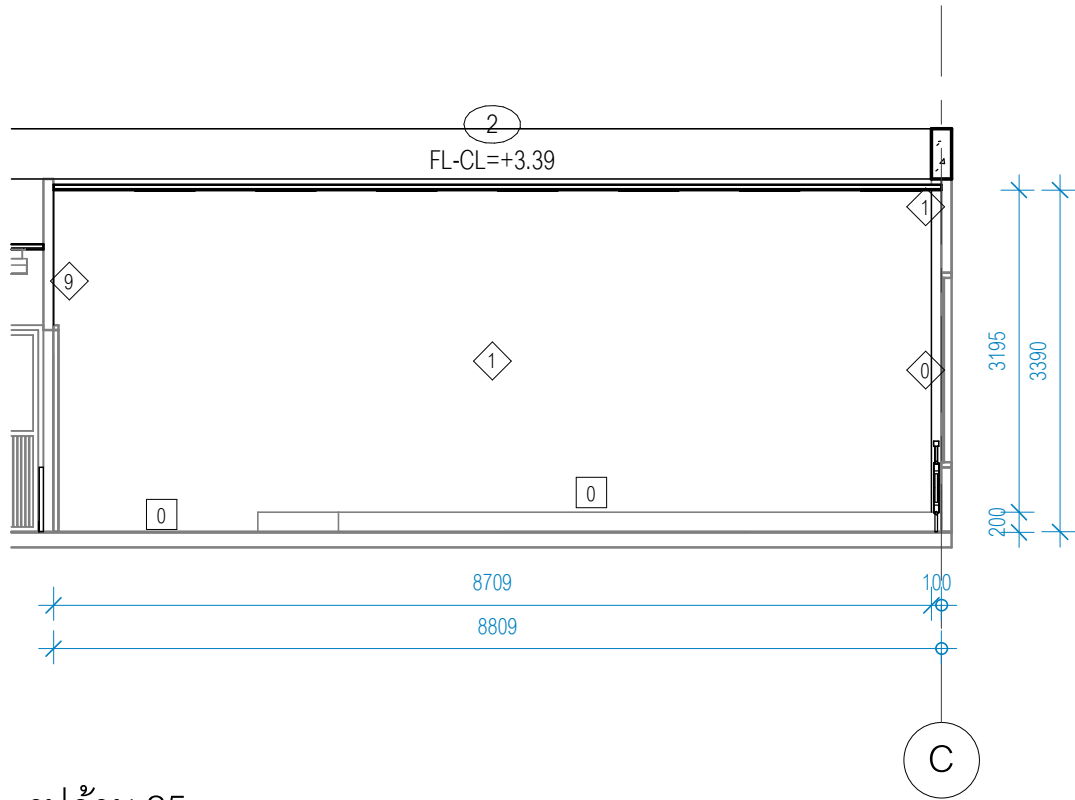
รูปด้าน 25
