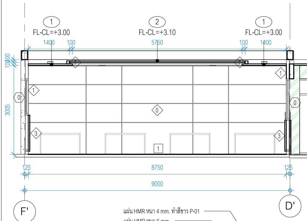
รูปด้าน 1 มาตราส่วน 1 : 75
