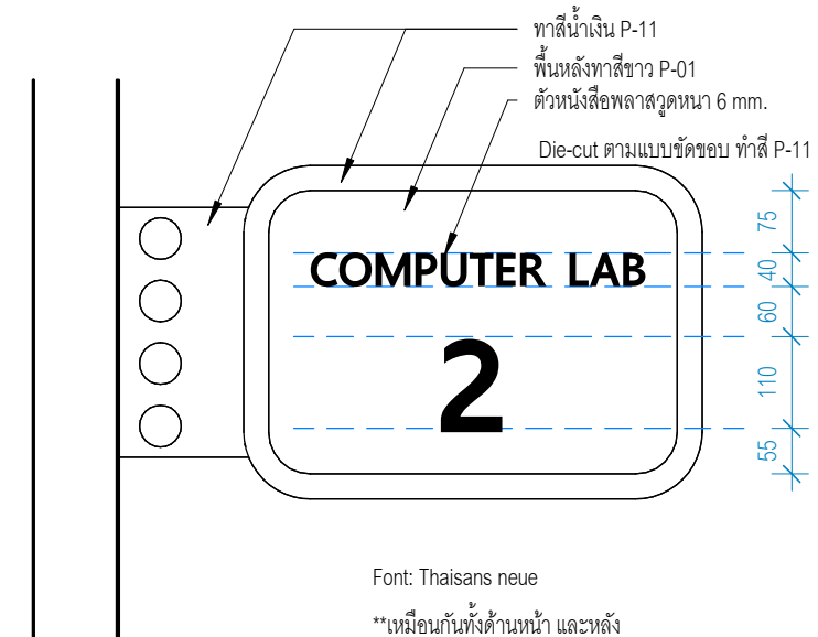
G-06 มาตรฐาน
