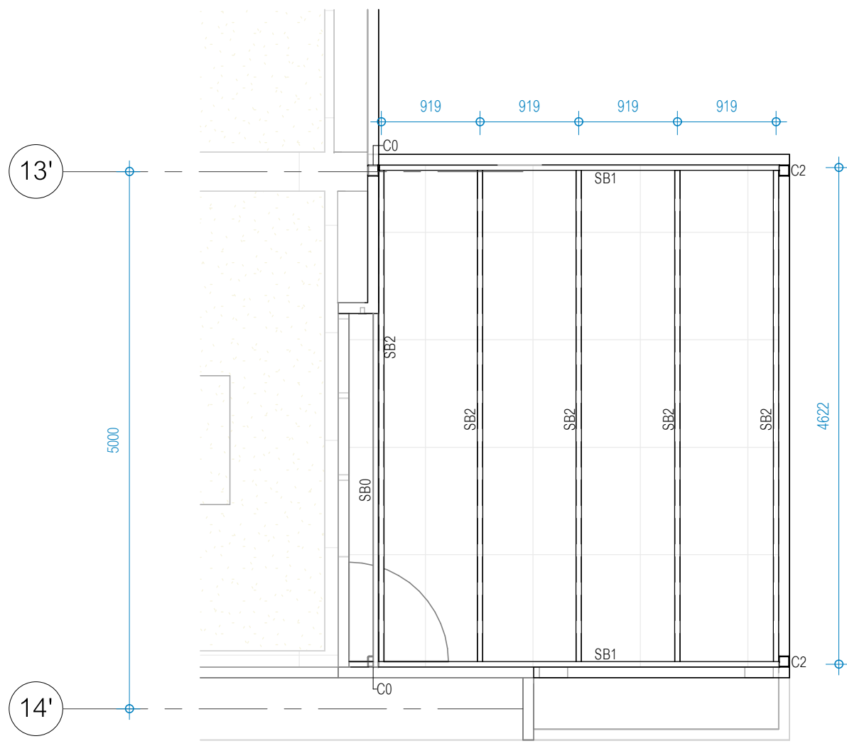
ผังโครงหลังคาส่วนต่อเติม มาตราส่วน 1 : 50
