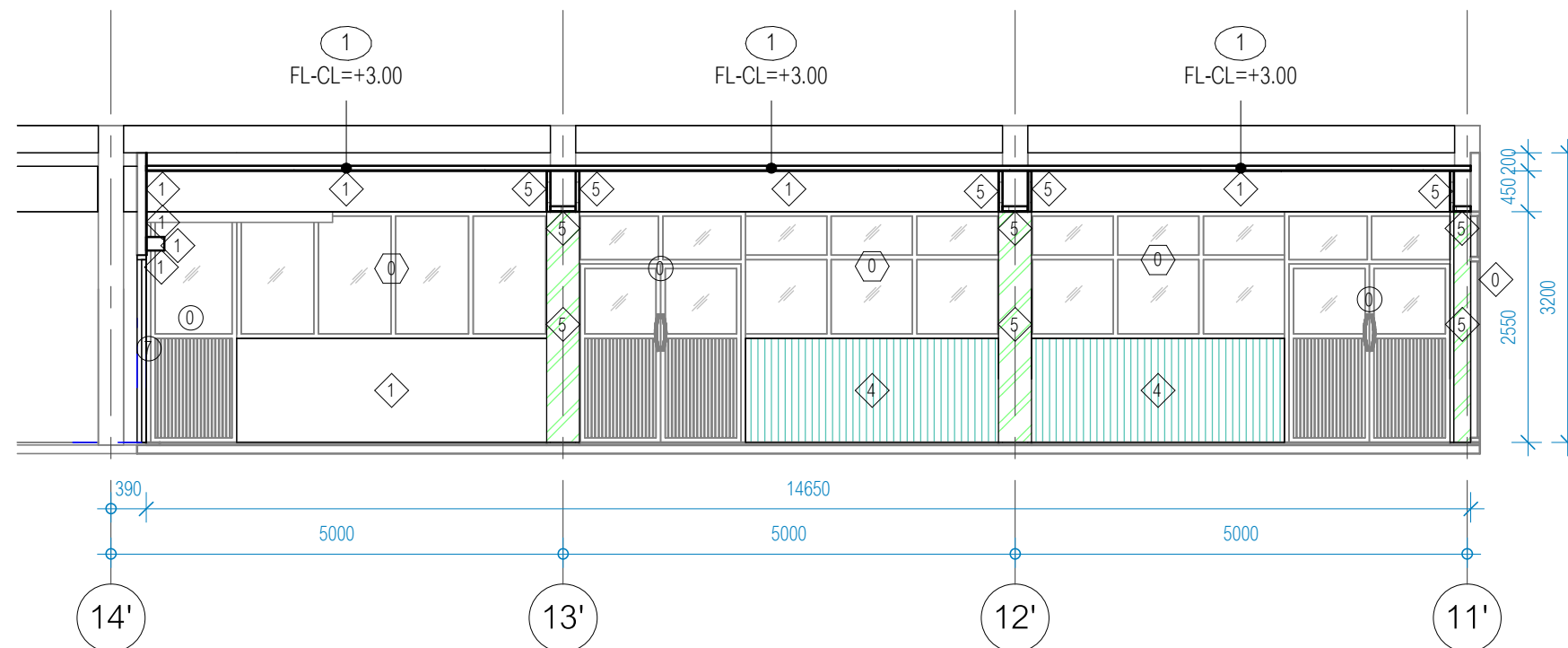
รูปด้าน 7
