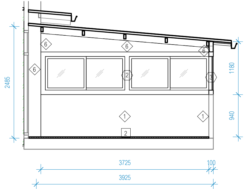
รูปด้าน 9 มาตราส่วน 1 : 50
