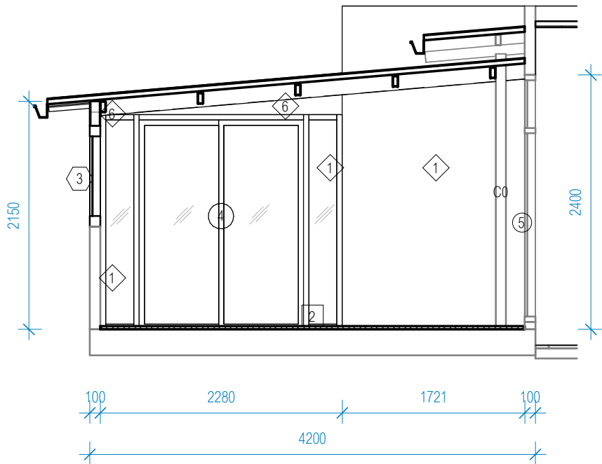
รูปด้าน 11 มาตราส่วน 1 : 50
