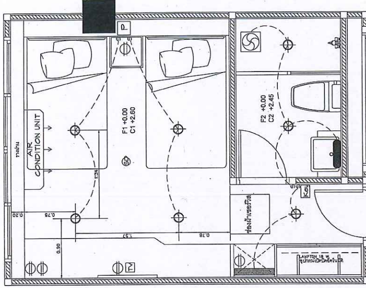
ไฟฟ้า-ห้องพัก PLAN-TWIN BEDDED ROOM The Suan Dusit Place Phase 1 - 5th floor
